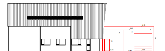
ALÇADO FRENTE
